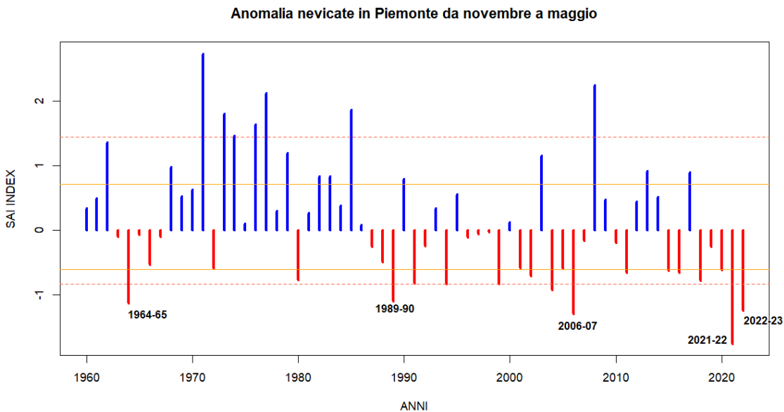
Figura 1: Indice di anomalia standardizzato della precipitazione nevosa in Piemonte (SAI - Standardized Anomaly Index) dal 1960 al 2022 basato sulla media del quarantennio 1981-2020. I valori delle stagioni che rimangono entro le linee continue (arancioni, che indicano rispettivamente il 1° e il 3° quartile) possono essere considerate nella media, mentre le variazioni che ricadono nell'intervallo tra le linee continue e quelle tratteggiate (rispettivamente nella parte negativa tra il 10° e il 25° percentile e nella parte positiva tra il 75° e il 90° percentile) sono considerate stagioni anomale, fuori dalla media. In ultimo le stagioni che ricadono al di sotto del 10° percentile e al di sopra del 90° percentile si considerano stagioni eccezionali.
