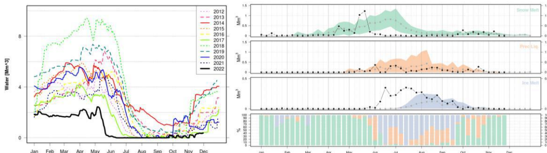
Figura 7: Risultati delle simulazioni sul bacino del Gabiet. Sinistra : evoluzione giornaliera dello swe per gli anni 2012-2022. Destra : andamento settimanale delle componenti del deflusso per l'anno 2022 in rapporto allo storico (2012-2021) delle simulazioni, dall'alto verso il basso: fusione nivale, pioggia, fusione glaciale, contributo percentuale di ciascuna componente al deflusso totale.
