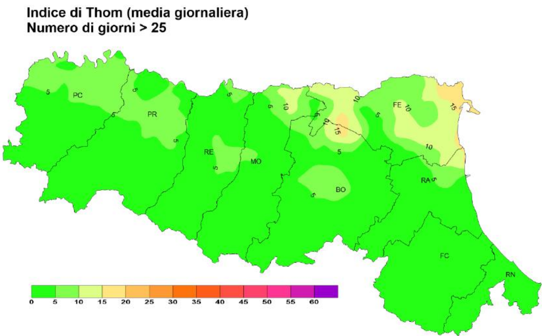
Figura 3: Mappa del numero di giorni dell'estate 2022 in cui l'indice di Thom è superiore a 25.
