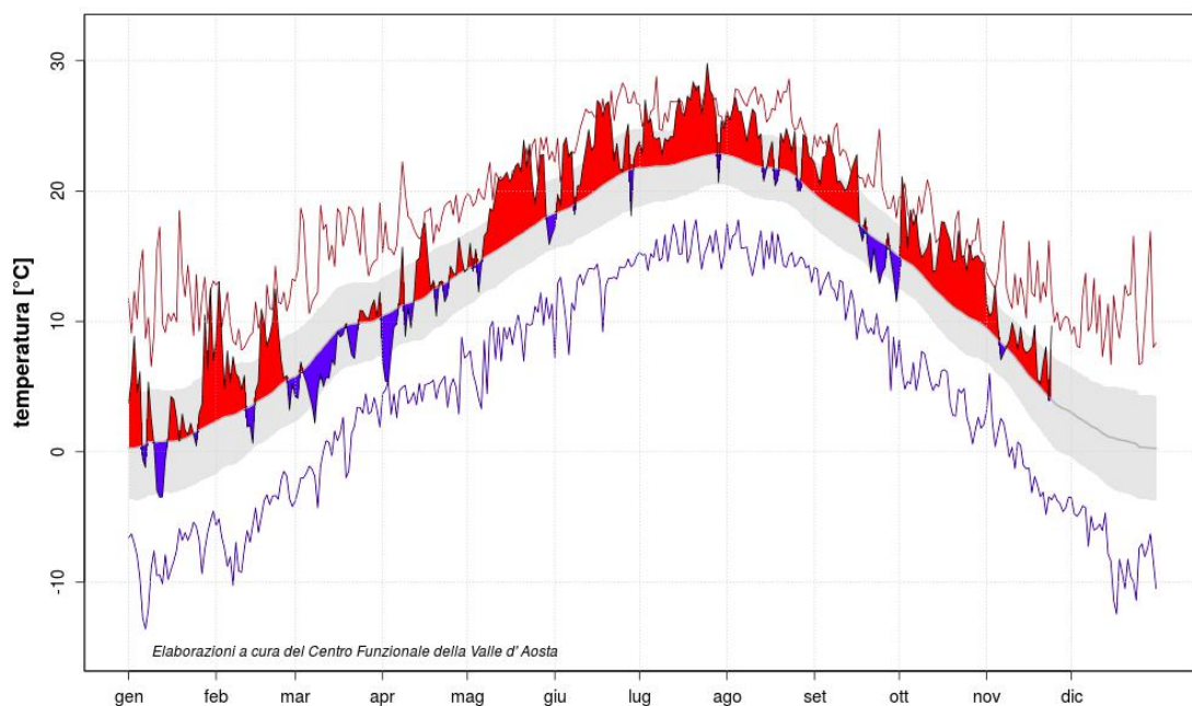
Figura 3: Andamento della temperatura media giornaliera nella piana di Aosta (Saint Christophe, a quota 550 m).
