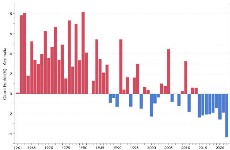
Figura 3.17: Serie delle anomalie medie annuali del numero di giorni freddi in Italia (TX10p) 7 , espresso in % di giorni/anno, rispetto al valore normale 1991-2020. Fonte: Elaborazione ISPRA.
