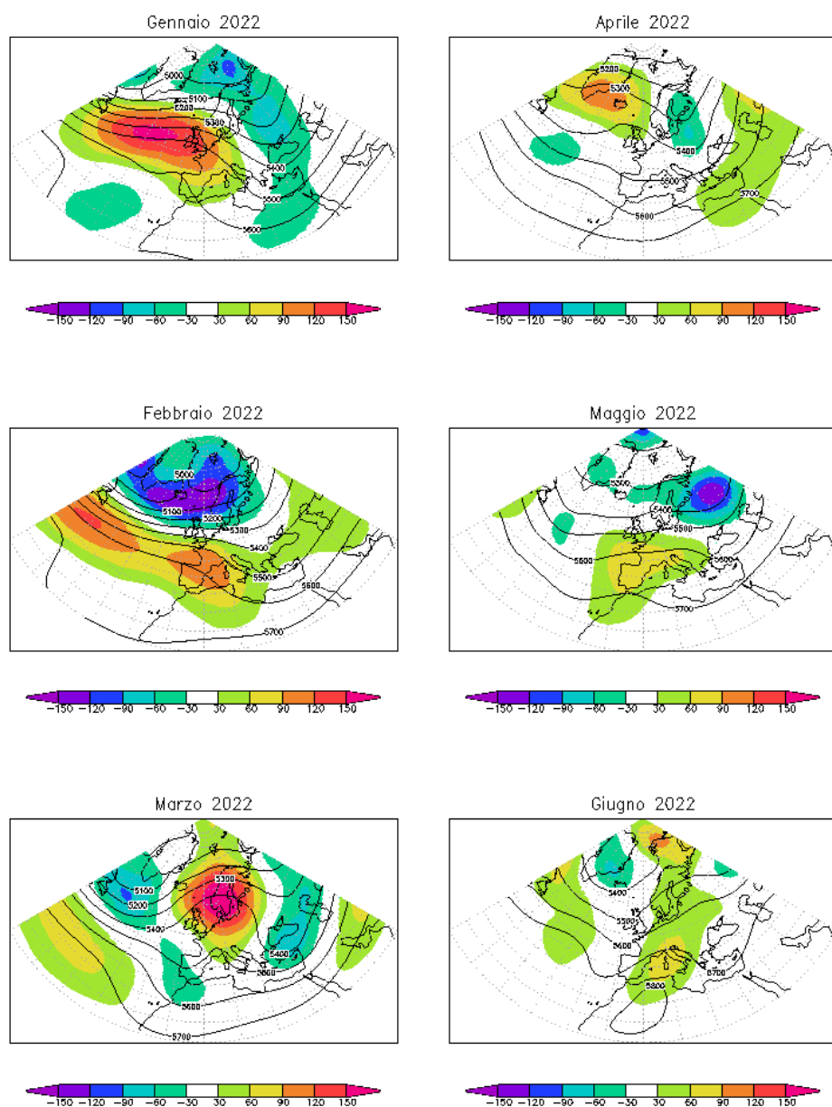
Figura 2.4a: Mappe del geopotenziale medio mensile (da gennaio a giugno 2022) a 500hPa. L'intervallo fra le isolinee è 100 mgs. Le aree colorate rappresentano l'anomalia 2022 rispetto al valore normale 1991-2020. Fonte: ERA5 - fifth generation ECMWF reanalysis, disponibile tramite la piattaforma del Copernicus Climate Change Service Copernicus.
