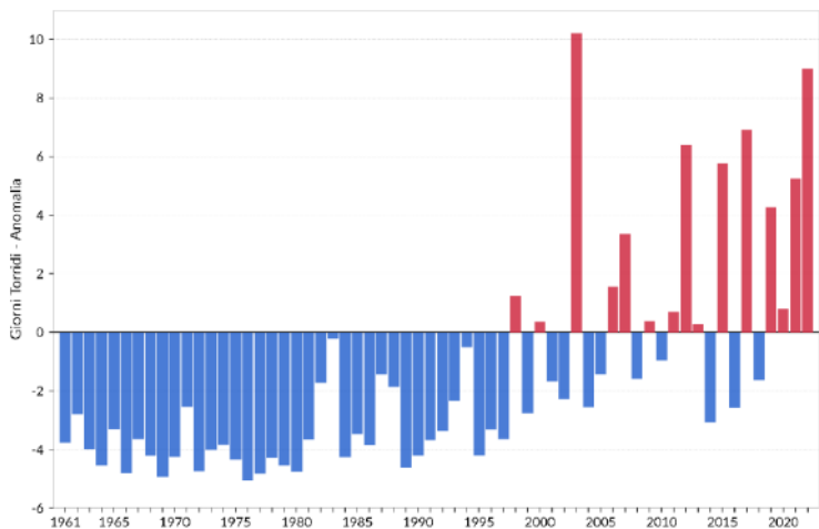
Figura 3.14: Serie delle anomalie medie annuali del numero di giorni torridi 4 in Italia rispetto al valore normale 1991-2020. Fonte: Elaborazione ISPRA.
