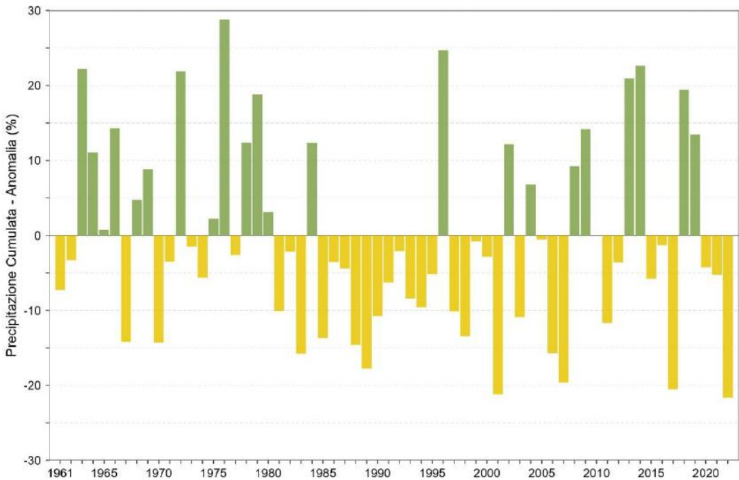
Figura 5.7: Serie delle anomalie medie in Italia, espresse in valori percentuali, della precipitazione cumulata annuale rispetto al valore normale 1991-2020. Fonte: Elaborazione ISPRA.
