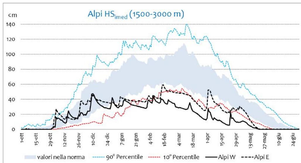
Figura 3: Andamento dello HS_{med} per le Alpi italiane nel trentennio 1991-2020, e per i settori W ed E delle Alpi italiane nella stagione invernale 2021-2022.
