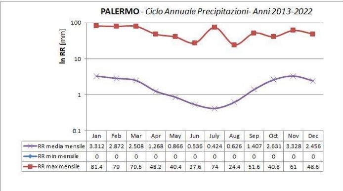
Figura 5: Ciclo annuale di precipitazioni (2013-2022).
