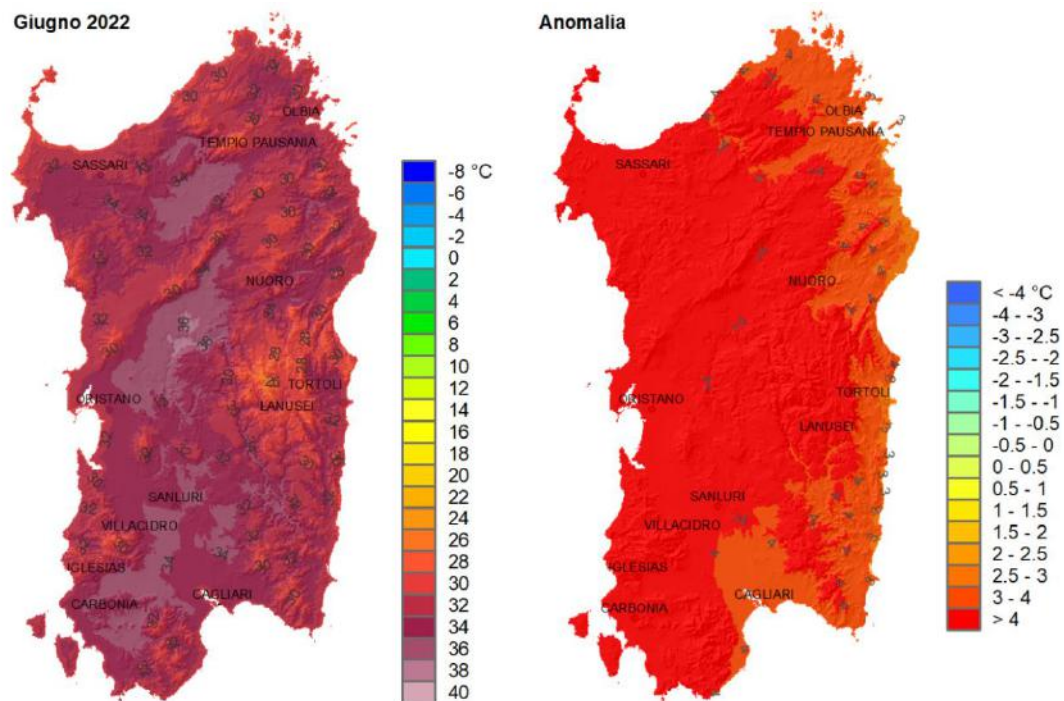
Figura 3: Valori medi mensili e anomalie climatiche delle temperature massime registrate nel mese di giugno 2022.
