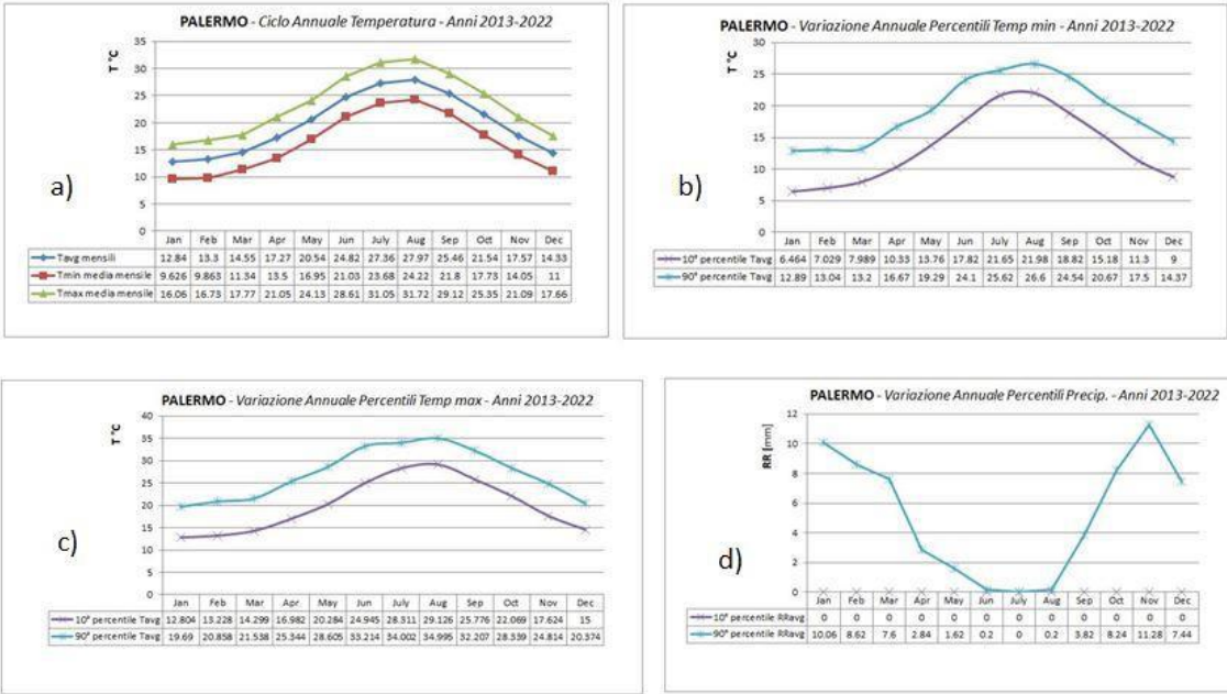
Figura 4: a) ciclo annuale di T; b) Variazione annuale percentili T minima; c) Variazione annuale percentili T massima; d) Variazione Annuale percentili precipitazione.
