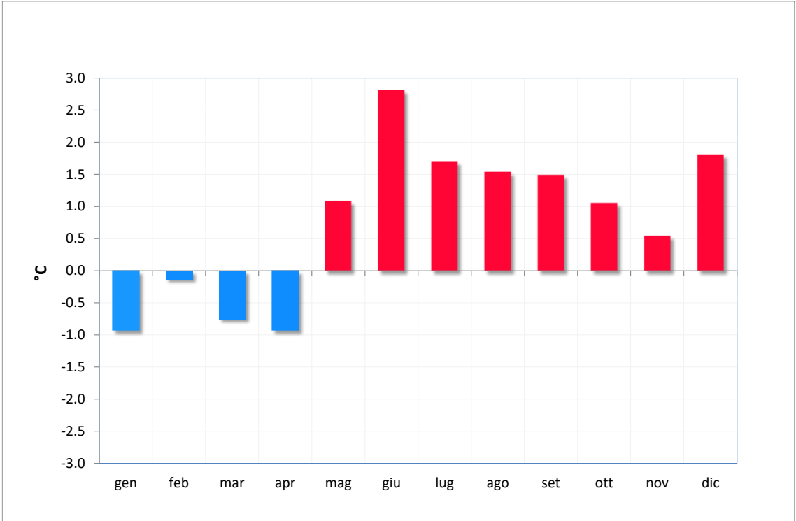
Figura 1: Anomalie climatiche delle Temperature minime 2022.
