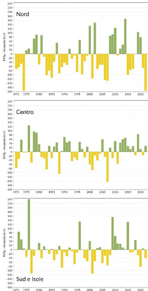
Figura 5.14: Serie delle anomalie medie al Nord, Centro, Sud e Isole, delle precipitazioni nei giorni molto piovosi (R95p) 11 , rispetto al valore normale 1991-2020. Fonte: Elaborazione ISPRA.
