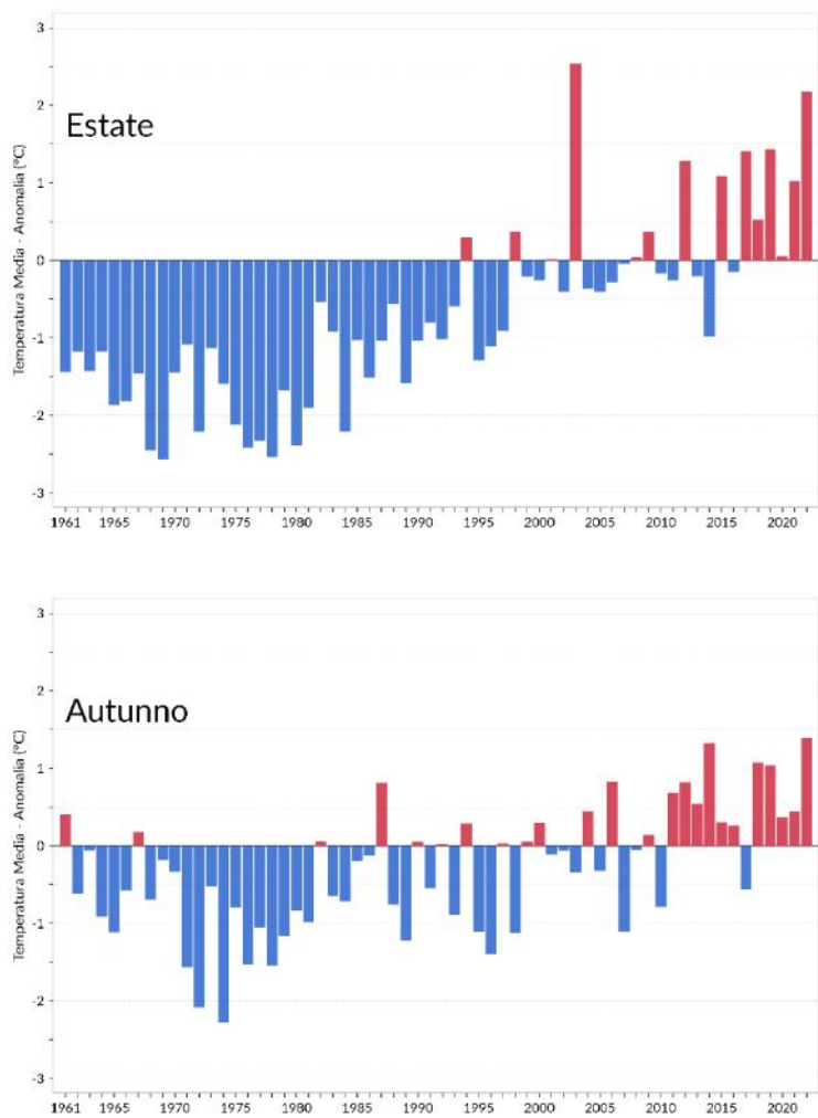
Figura 3.10b: Serie delle anomalie medie stagionali della temperatura media in Italia rispetto al valore normale 1991-2020 (estate e autunno). Fonte: Elaborazione ISPRA.
