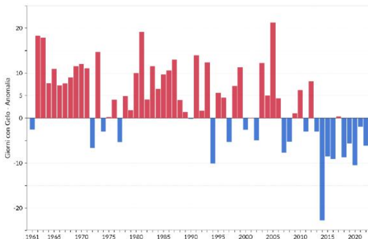
Figura 3.11: Serie delle anomalie medie annuali del numero di giorni con gelo 1 in Italia rispetto al valore normale 1991-2020. Fonte: Elaborazione ISPRA.
