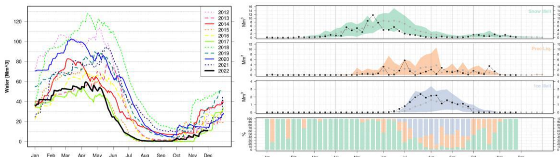
Figura 6: Risultati delle simulazioni sul bacino di Place Moulin. Sinistra : evoluzione giornaliera dello swe per gli anni 2012-2022. Destra : andamento settimanale delle componenti del deflusso per l'anno 2022 in rapporto allo storico (2012-2021) delle simulazioni, dall'alto verso il basso: fusione nivale, pioggia, fusione glaciale, contributo percentuale di ciascuna componente al deflusso totale.
